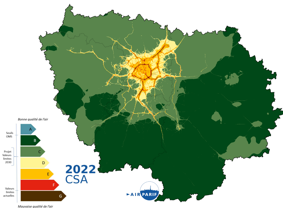
La carte stratégique de la qualité de l'air obtenue pour l'année 2022 pour la région Île-de-France (source : Airparif).
